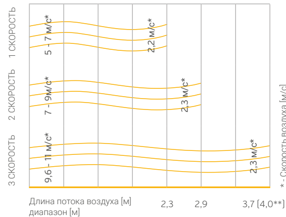
Длина горизонтальной струи воздуха (при вертикальном монтаже)
